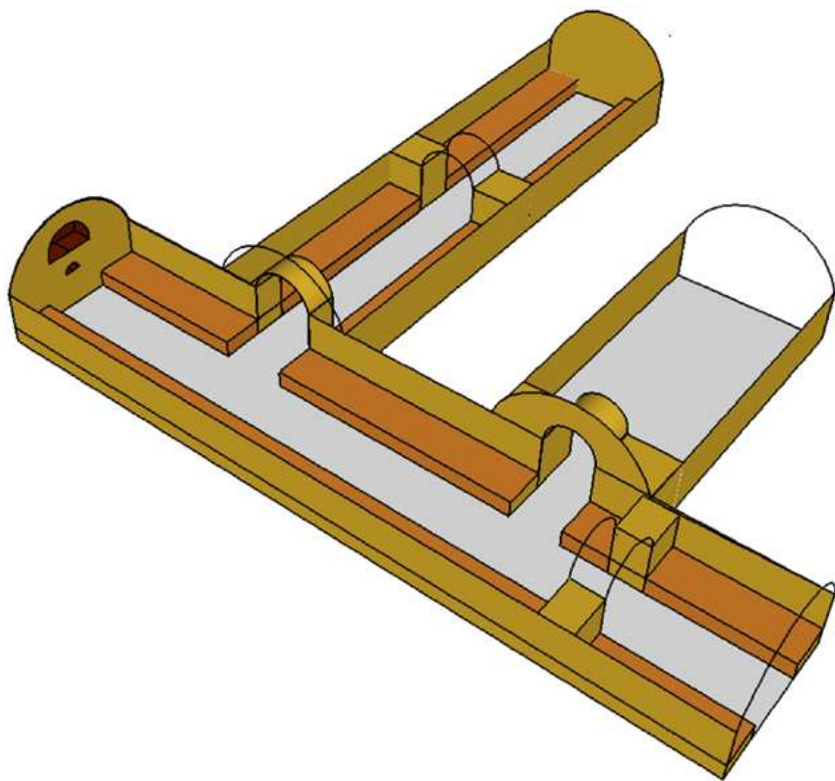
Figura 31.- Restitució 3D del refugi de la Plaça de la Creu. (El·laboració pròpia).
